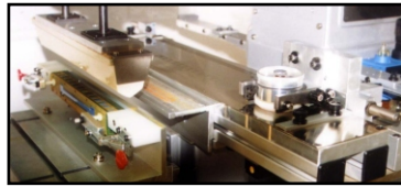
- Tintero lateral para la impresión de imágenes largas (SCMIC).
